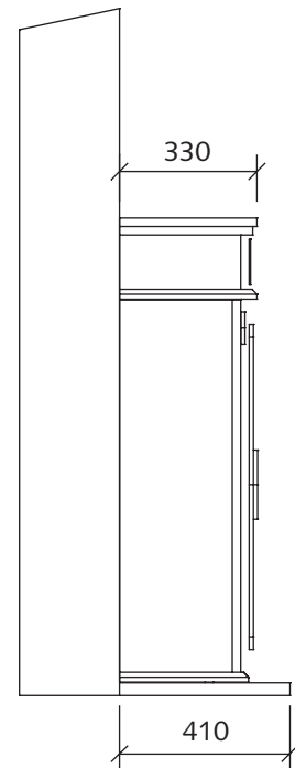
Seitenansicht
