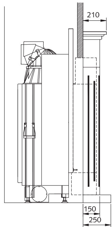
Seitenansicht
