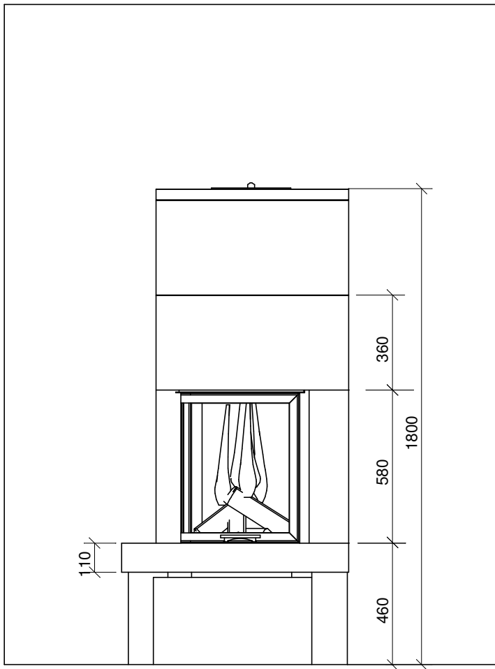
Ansicht
